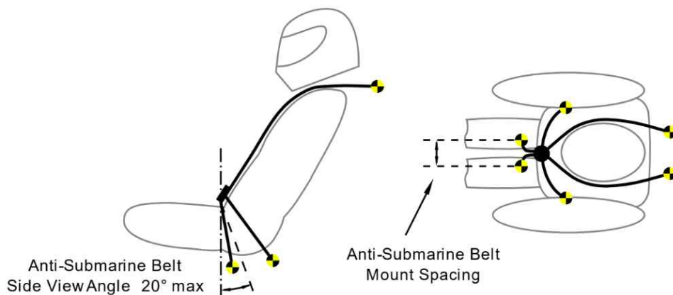
그림 22. 다리사이 벨트 조건
