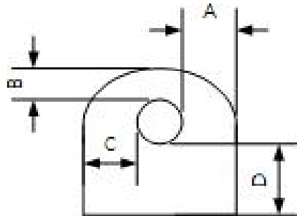
그림18. 벨트 마운트 브라켓
