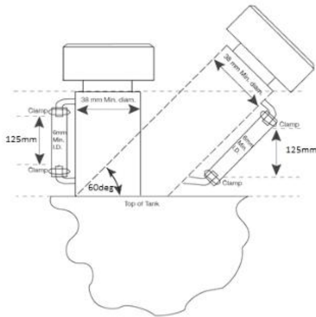
그림28. 연료통 주입 연료량 확인 조건
