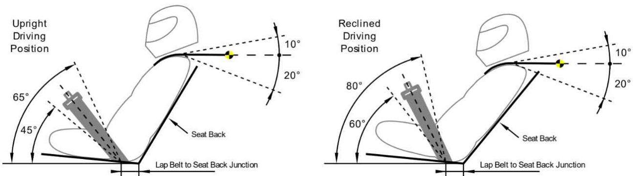
그림 20. 허리벨트 조건
