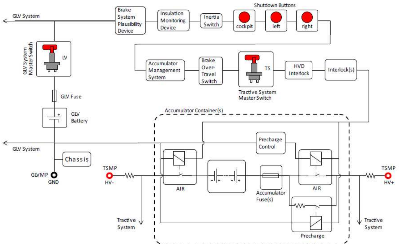
그림36. 차단 회로
