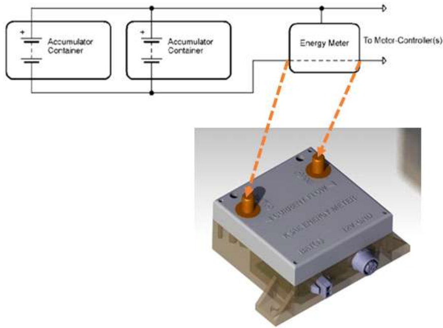
그림39. 에너지미터 연결 개략도
