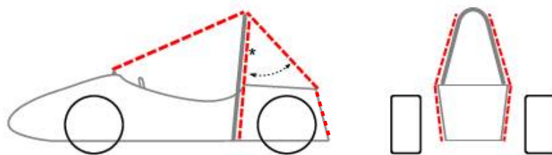
그림33. 롤오버 보호 영역
