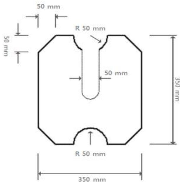
그림6. 운전석 단면 확인용 측정도구
