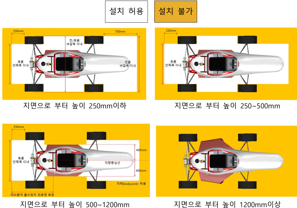
그림 42. 공력장치
