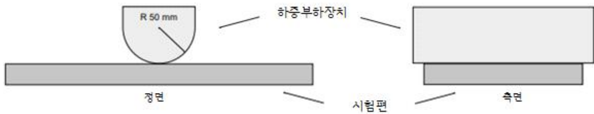
그림17. 복합재 테스트
