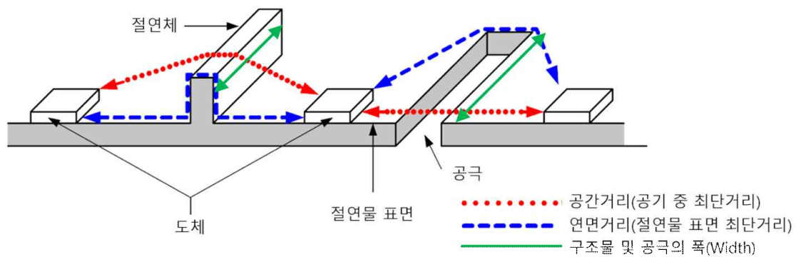
그림32. 절연
