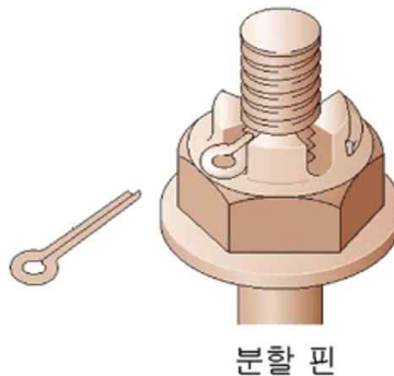
그림.0 허브센터 볼트 풀림방지 적용 예시
