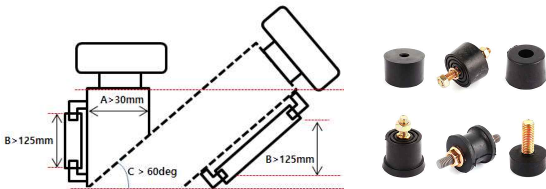
그림13. 연료주입구와 연료량표시기의 조건과 방진고무볼트
