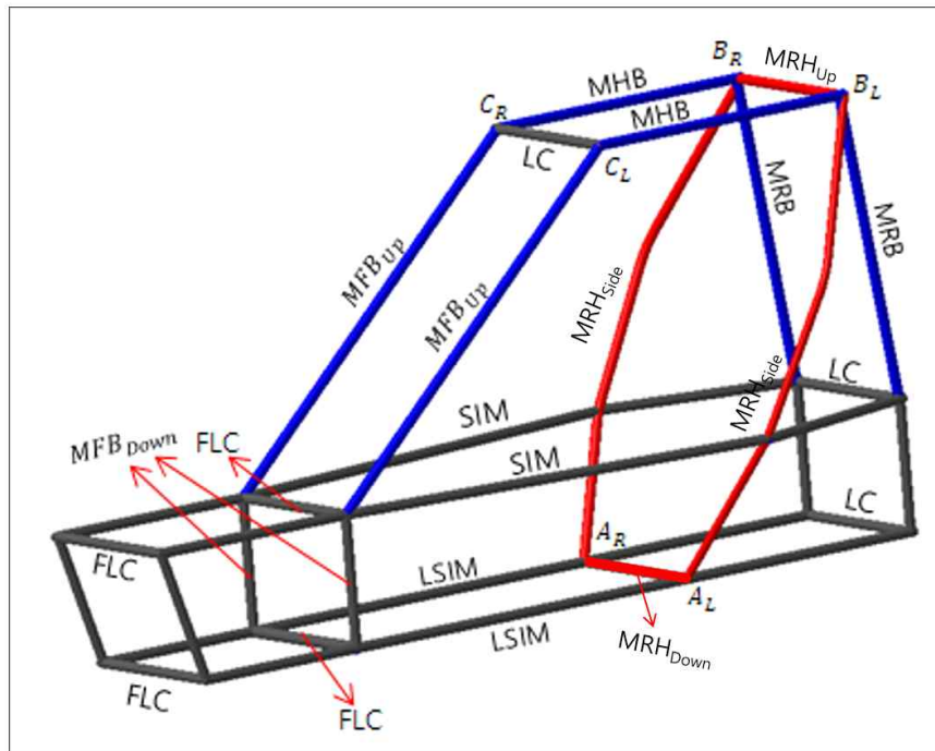
그림1. 롤 케이지
