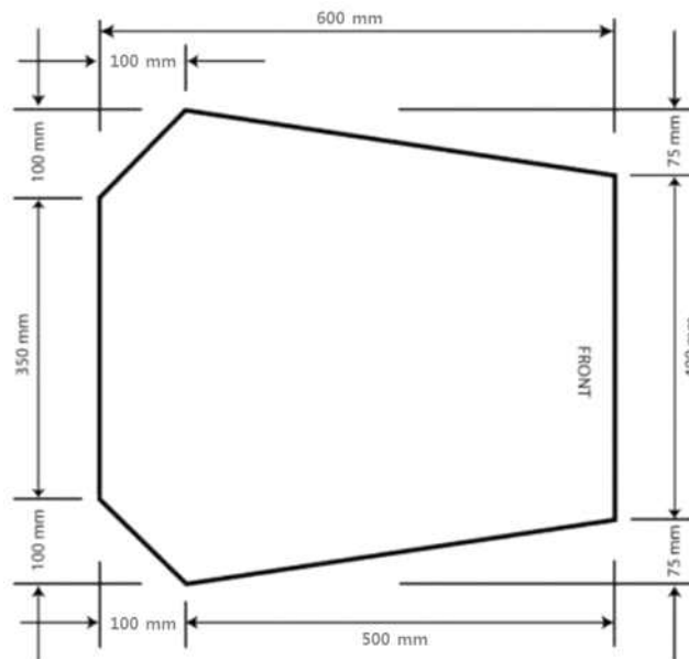
그림5. 운전석 공간 확인용 측정도구
