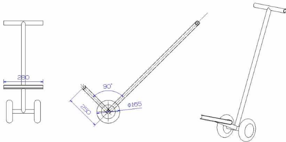
그림 44. 퀵 잭(Quick Jack) 예
