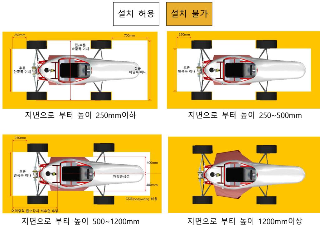
그림 42. 공력장치
