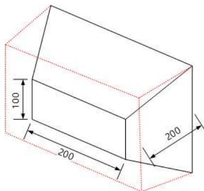
그림 15. 충격완화장치 예시
