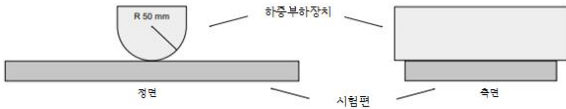
그림17. 복합재 테스트
