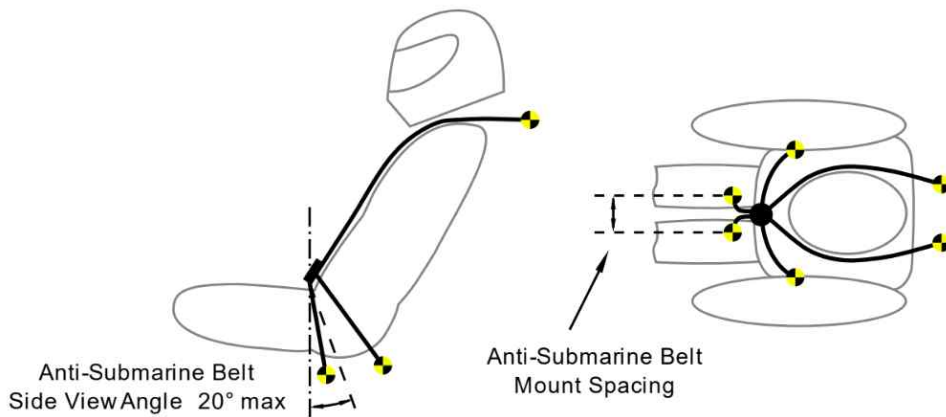
그림21. 다리사이 벨트 조건
