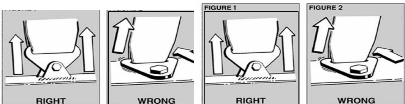
그림18. 벨트 설치 예
