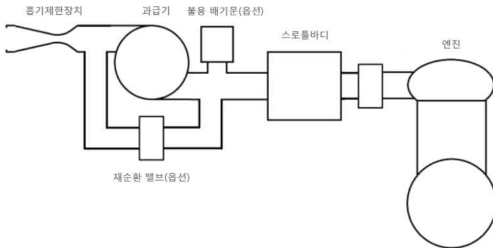
그림 25. 과급기 사용 시 흡기제한장치 위치
