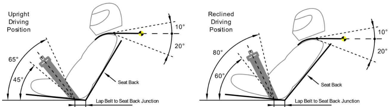
그림19. 허리벨트 조건
