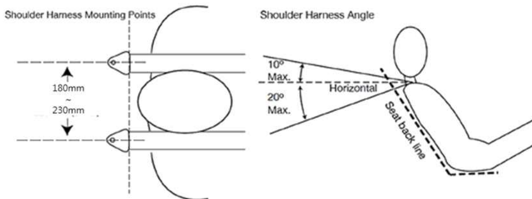
그림20. 어깨벨트 조건
