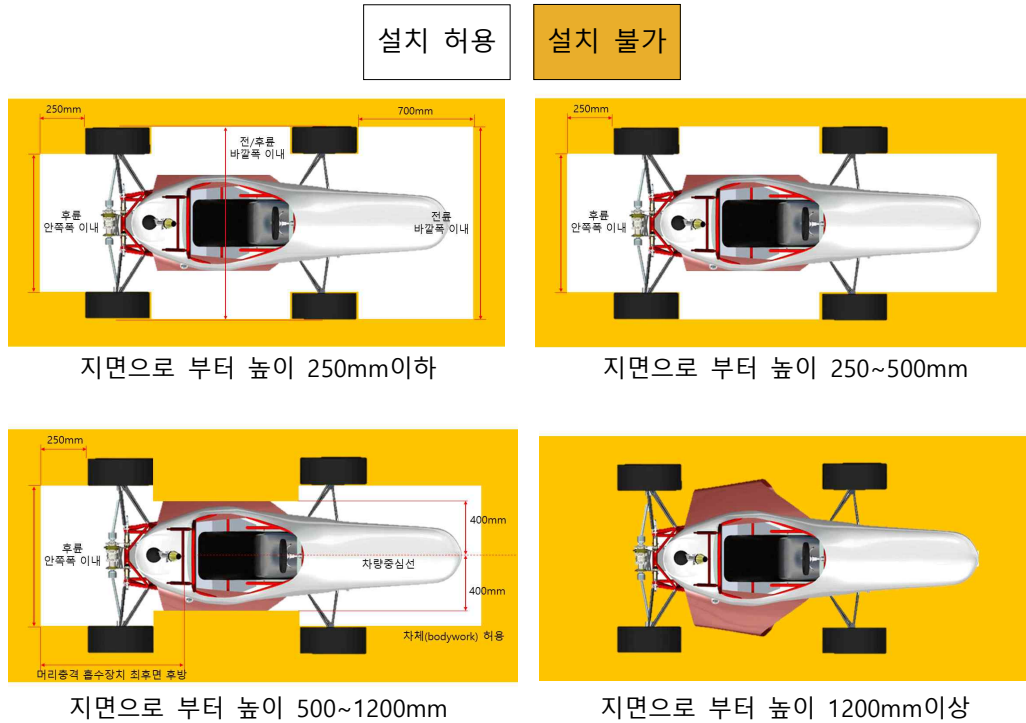
그림40. 공력장치
