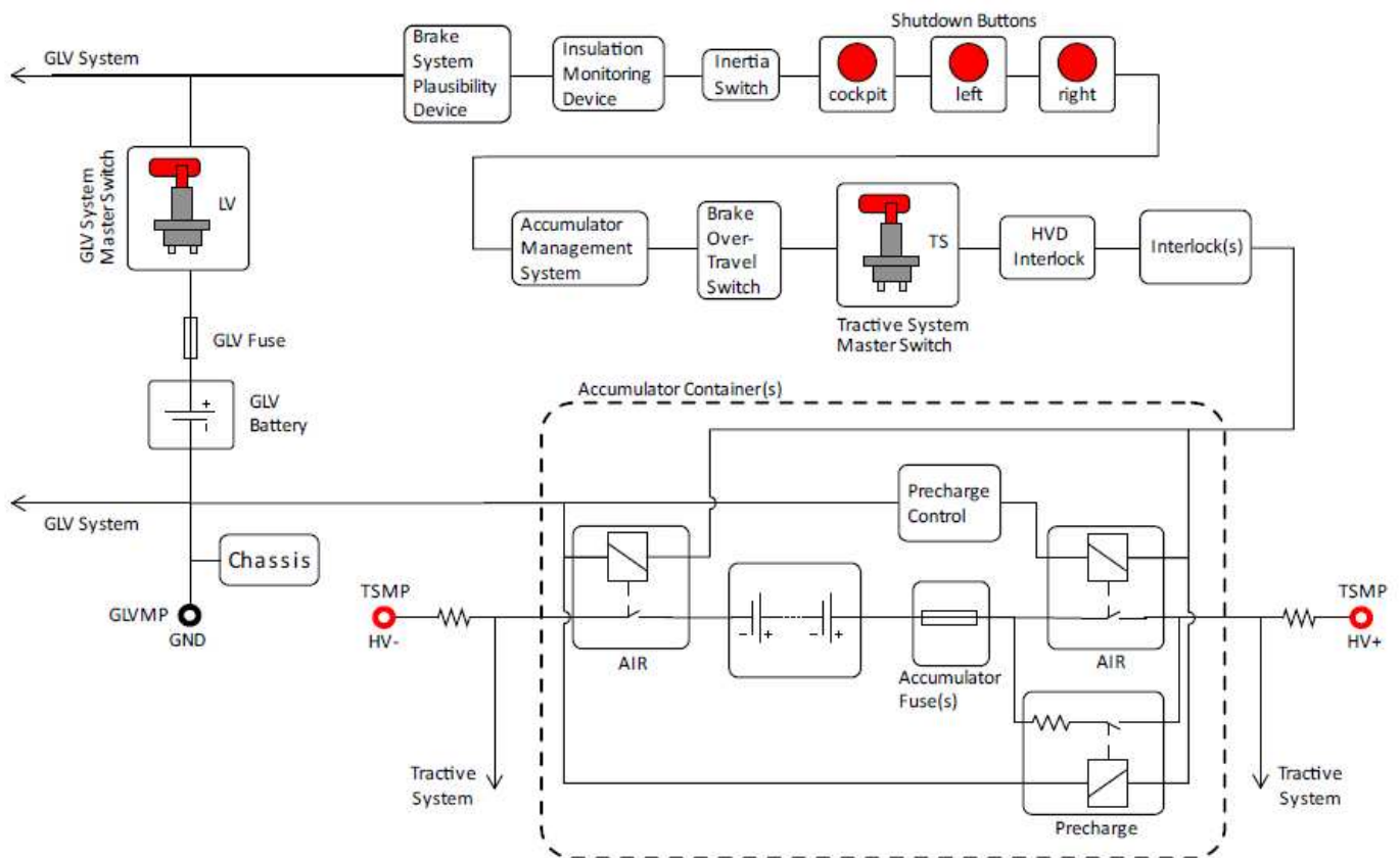
그림36. 차단 회로
