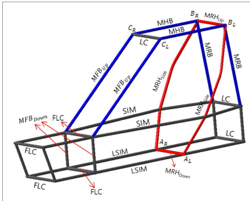
그림1. 롤 케이지
