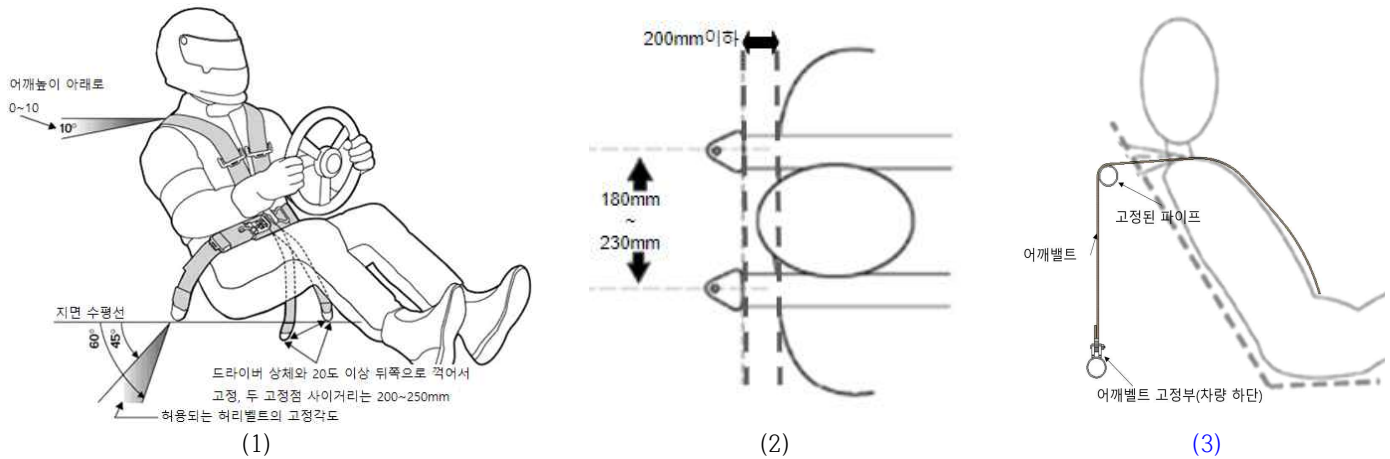
그림4. 벨트장착의 예
