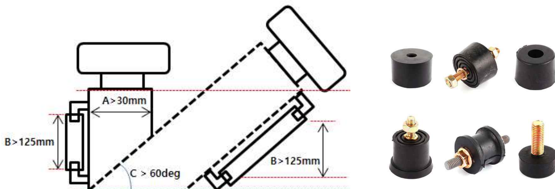
그림 13. 연료주입구와 연료량표시장치의 조건과 방진고무볼트
