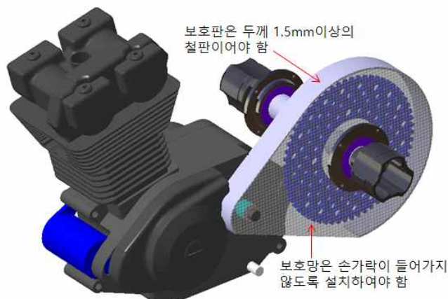
그림10. 보호판 및 보호망
