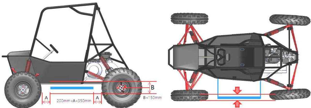
그림2. 측면범퍼 설치 예시
