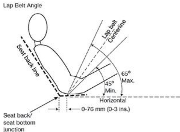
그림19. 허리벨트 조건
