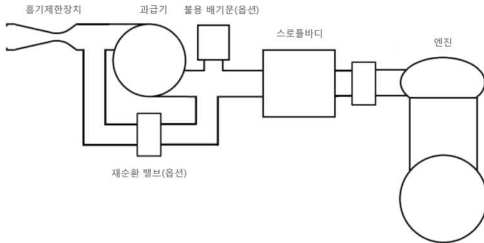
그림 24. 과급기 사용 시 흡기제한장치 위치
