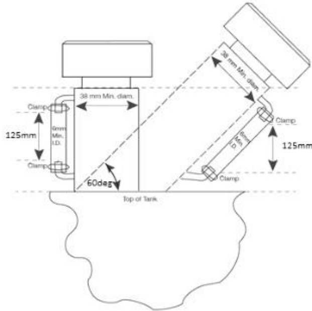
그림26. 연료통 주입 연료량 확인 조건
