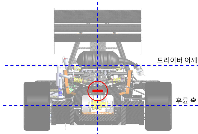
그림2. 제동등 위치
