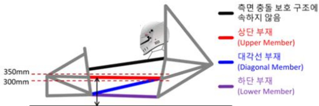
그림16. 측면 충돌 보호 구조물 정의 및 조건
