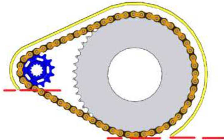
그림 25. 구동 장치 보호판의 끝부분
