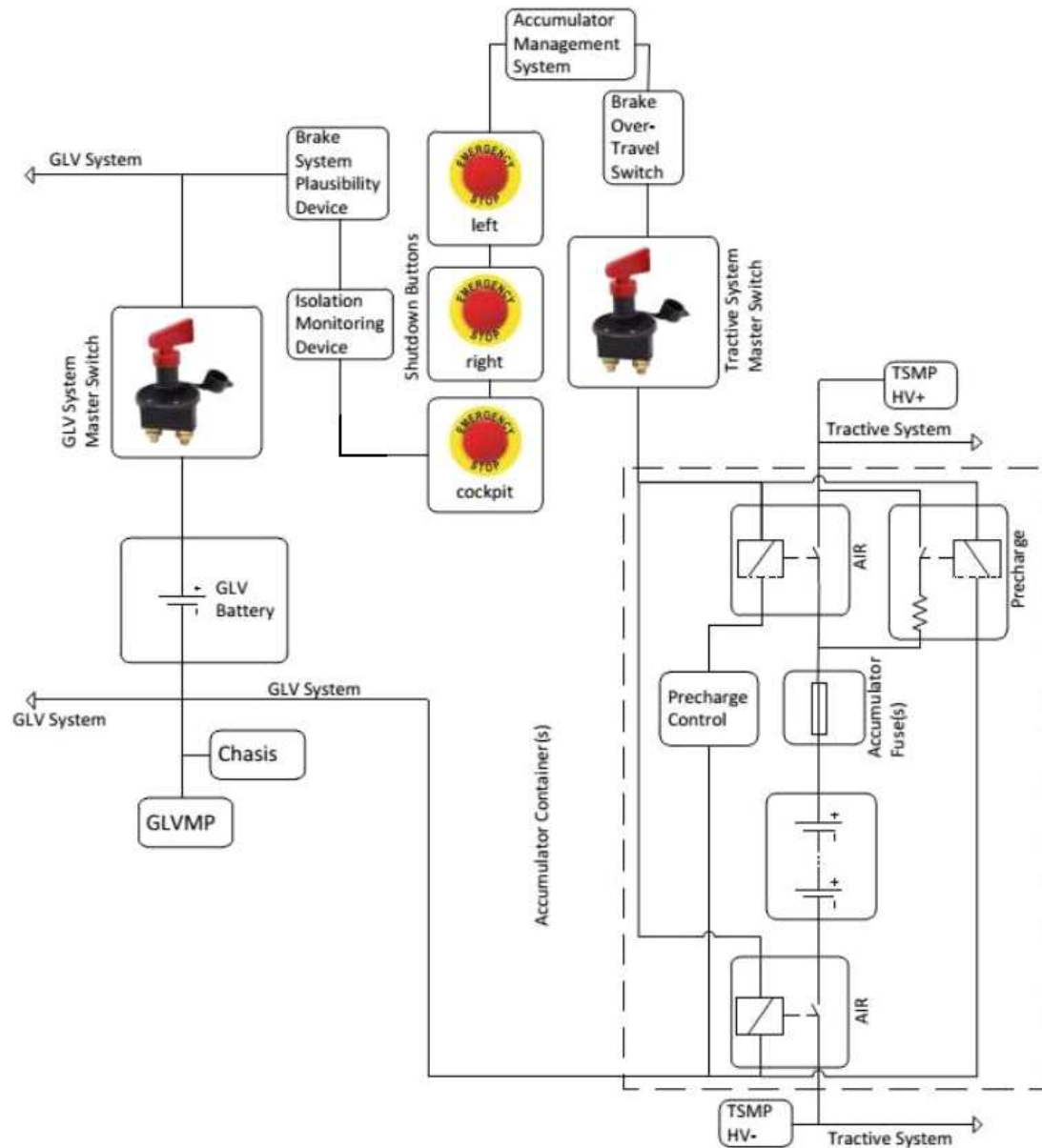
그림33. 차단 회로
