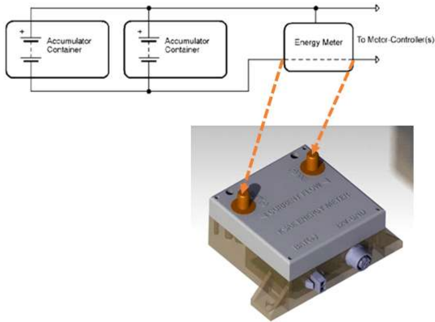
그림35. 에너지미터 연결 개략도
