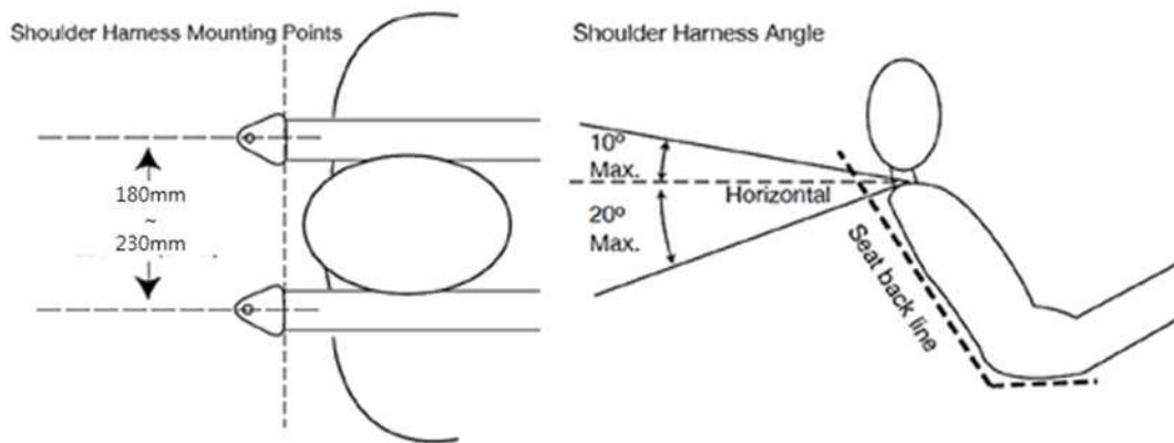
그림20. 어깨벨트 조건
