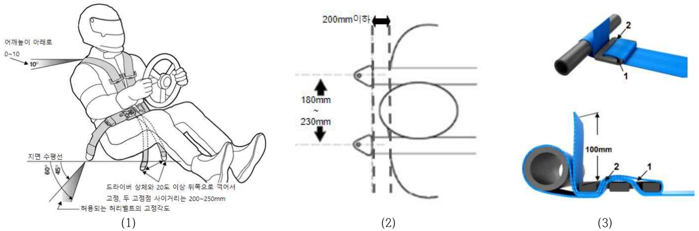
그림4. 벨트장착의 예
