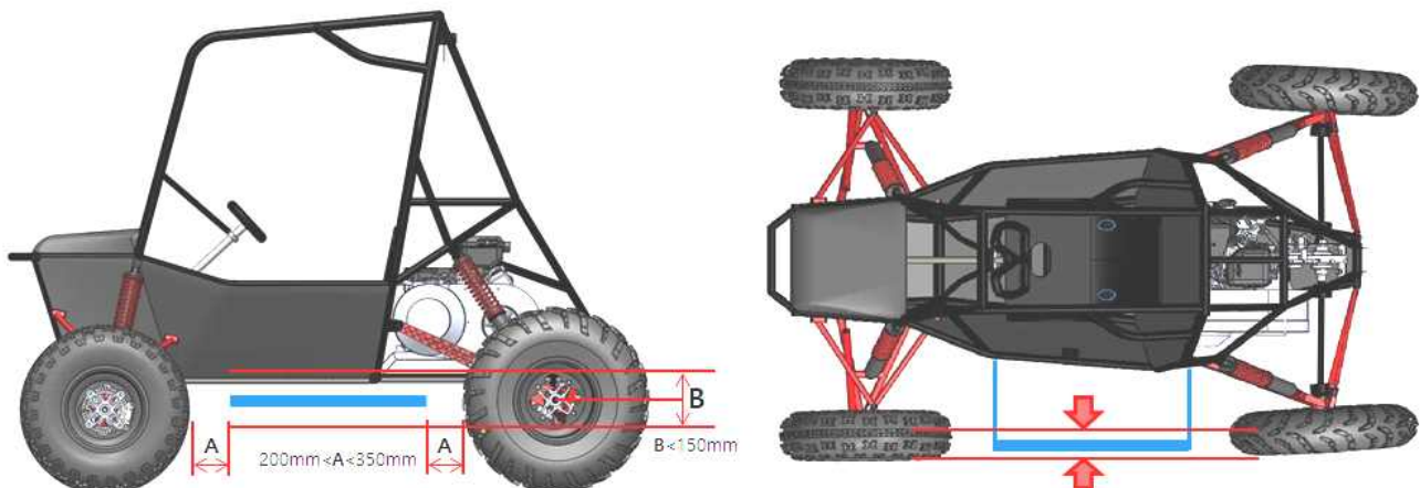
그림2. 측면범퍼 설치 예시
