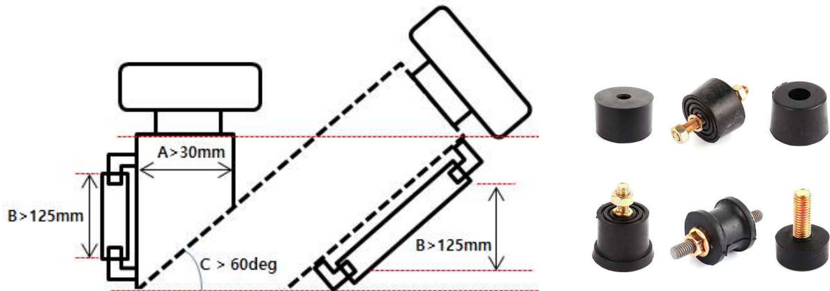
그림 13. 연료주입구와 연료량표시기의 조건과 방진고무볼트
