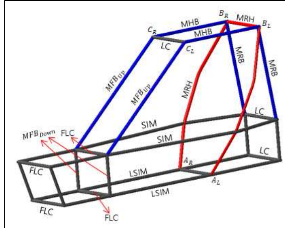
그림1. 롤 케이지
