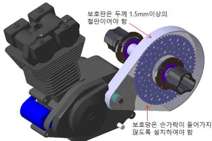
그림 10. 보호판 및 보호망
