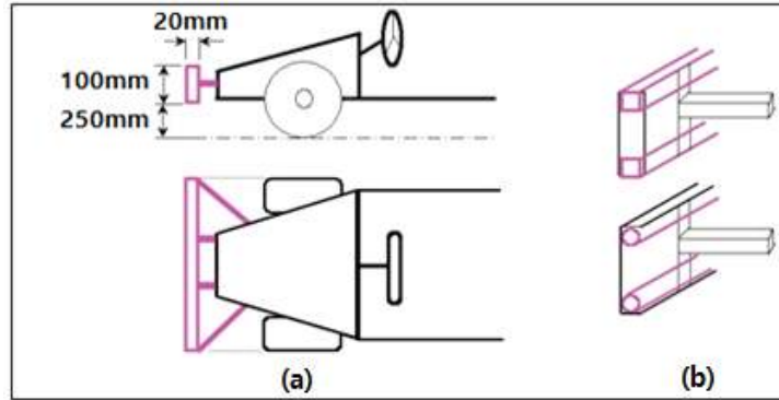
그림5. 범퍼 설치도 및 범퍼 단면도
