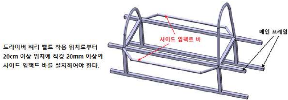
그림2. 사이드 임팩트 설치 예
