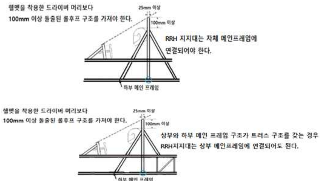
그림3. 롤 후프 및 롤 후프 지지대 설치 예
