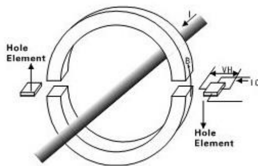
그림34. 에너지미터 연결
