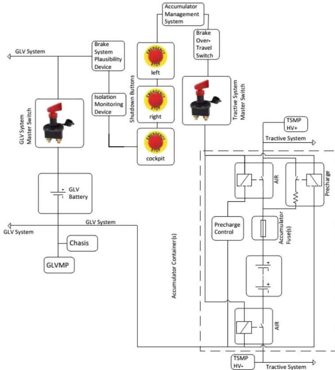
그림32. 차단 회로
