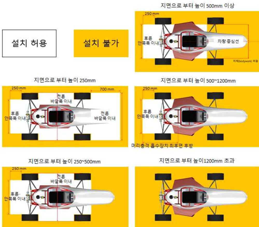
그림39. 공력장치
