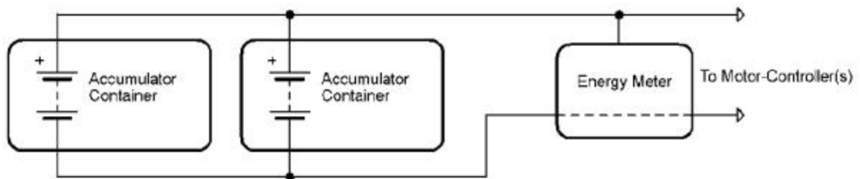
그림35. 에너지미터 연결 개략도
