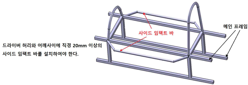
그림 2. 사이드 임팩트 설치 예
