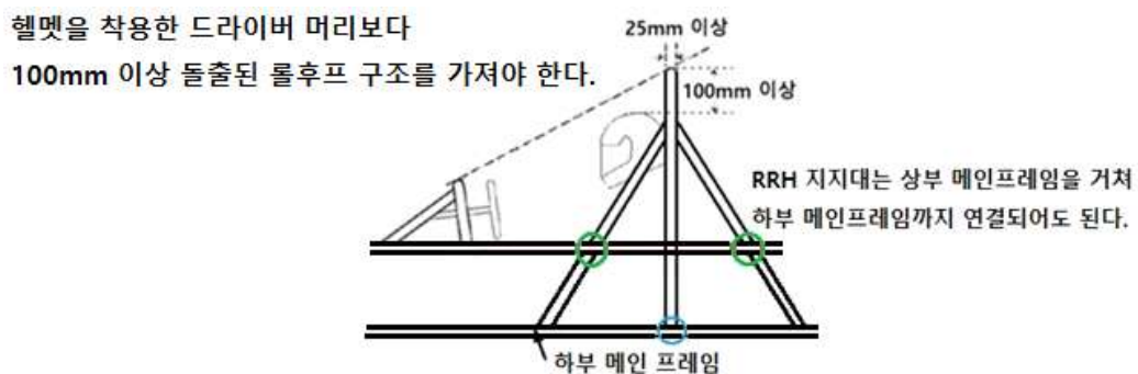
그림 3. 사이드 임팩트 바 및 롤 후프 구조 예
