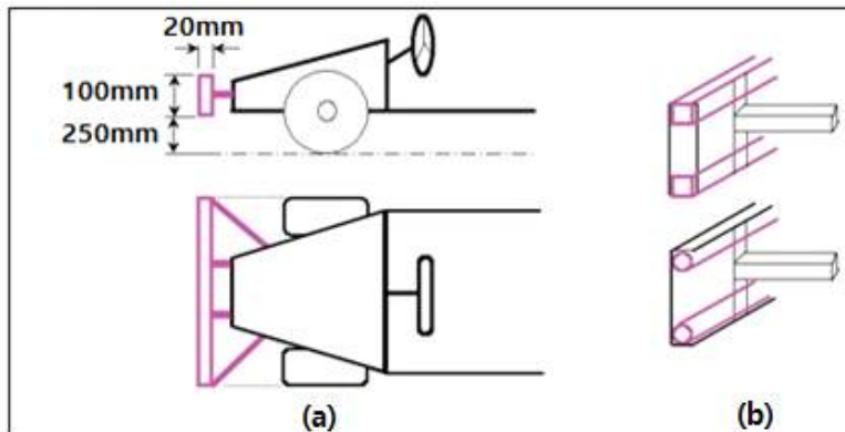
그림5. 범퍼 설치도 및 범퍼 단면도
